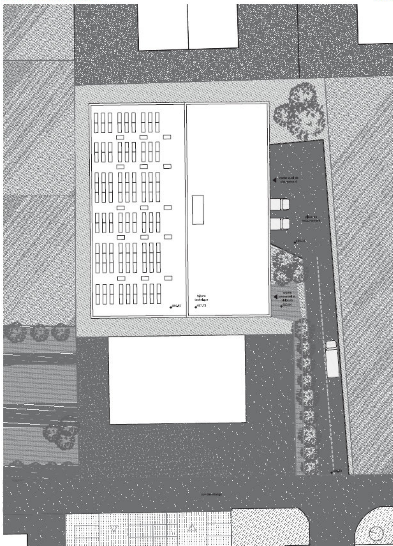
Plan de situation 1:200
