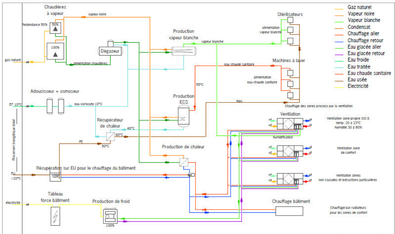
schéma réseaux techniques
