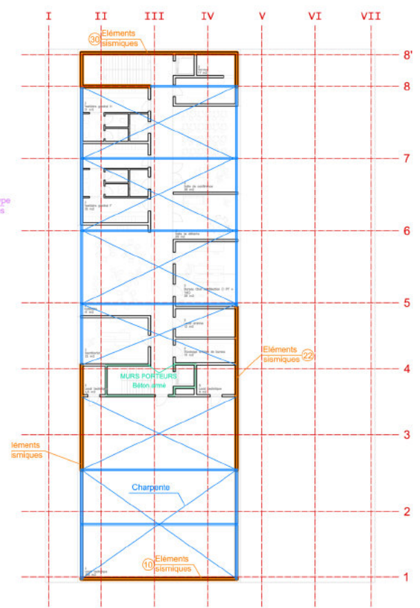
Plan structurel de l'étage
