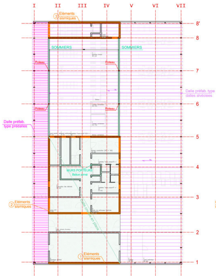
Plan structurel du rez
